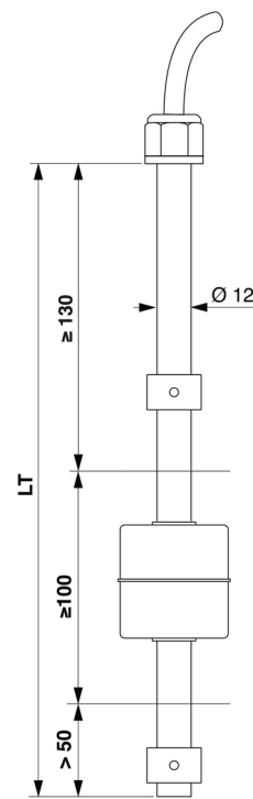
Salida cable
