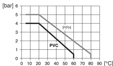
Presión vs. Temperatura
